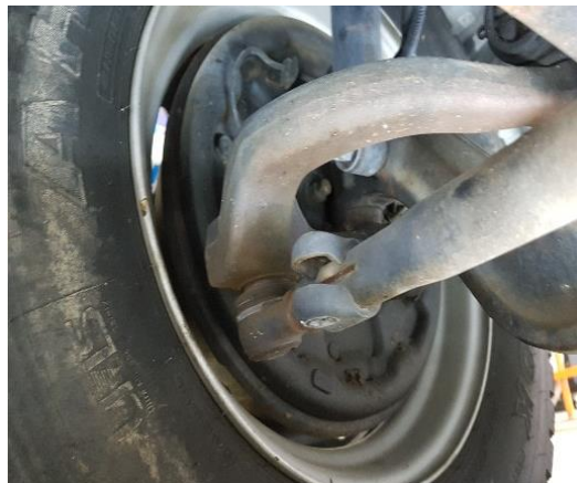
타이로드 엔드 설치상태 불량
