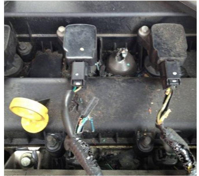
인젝터 배선 손상
